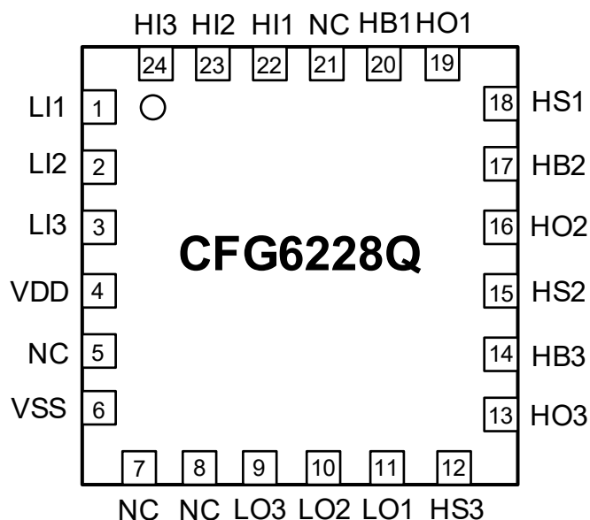
图5-1 封装引脚图
