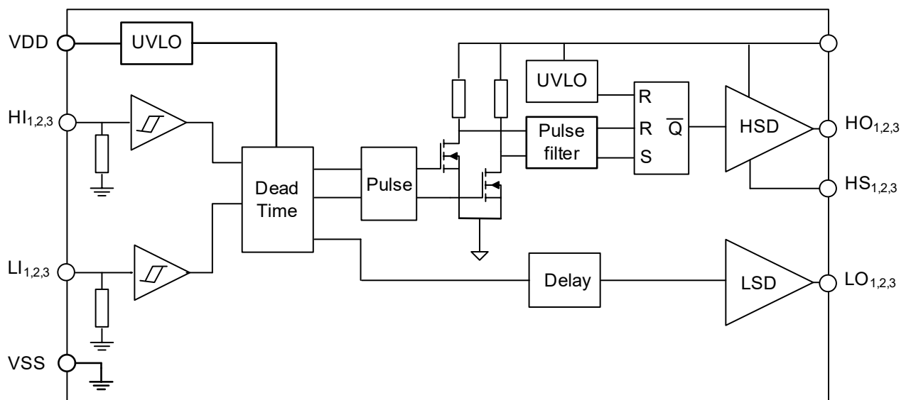
内部框图
