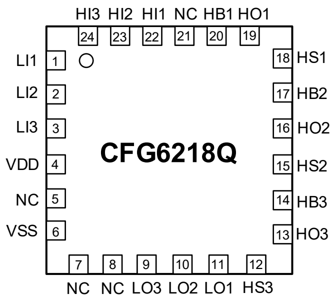
图5-2 封装引脚图
