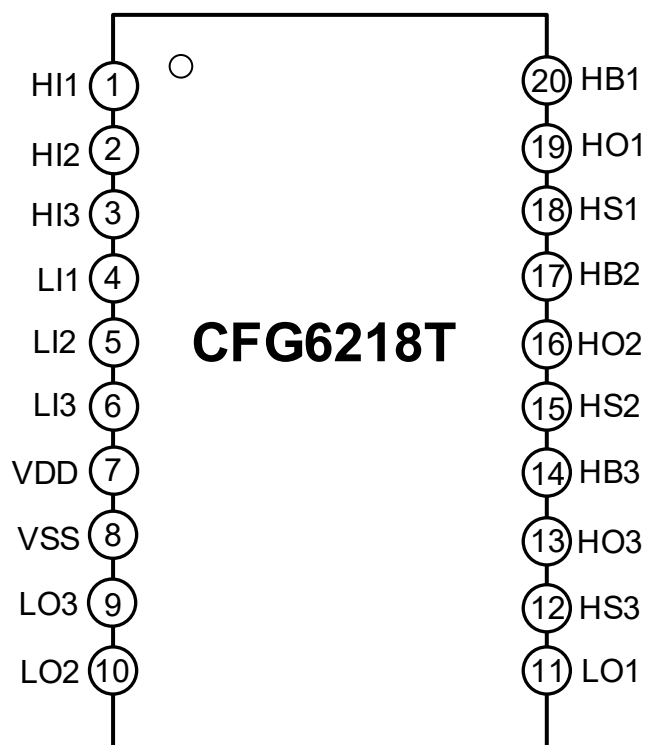
图5-1 封装引脚图
