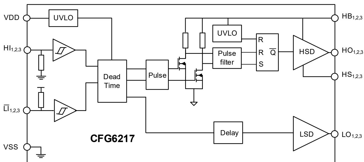
内部框图
