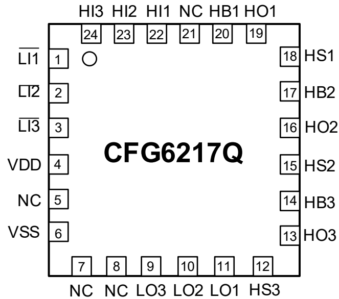
图5-2 封装引脚图
