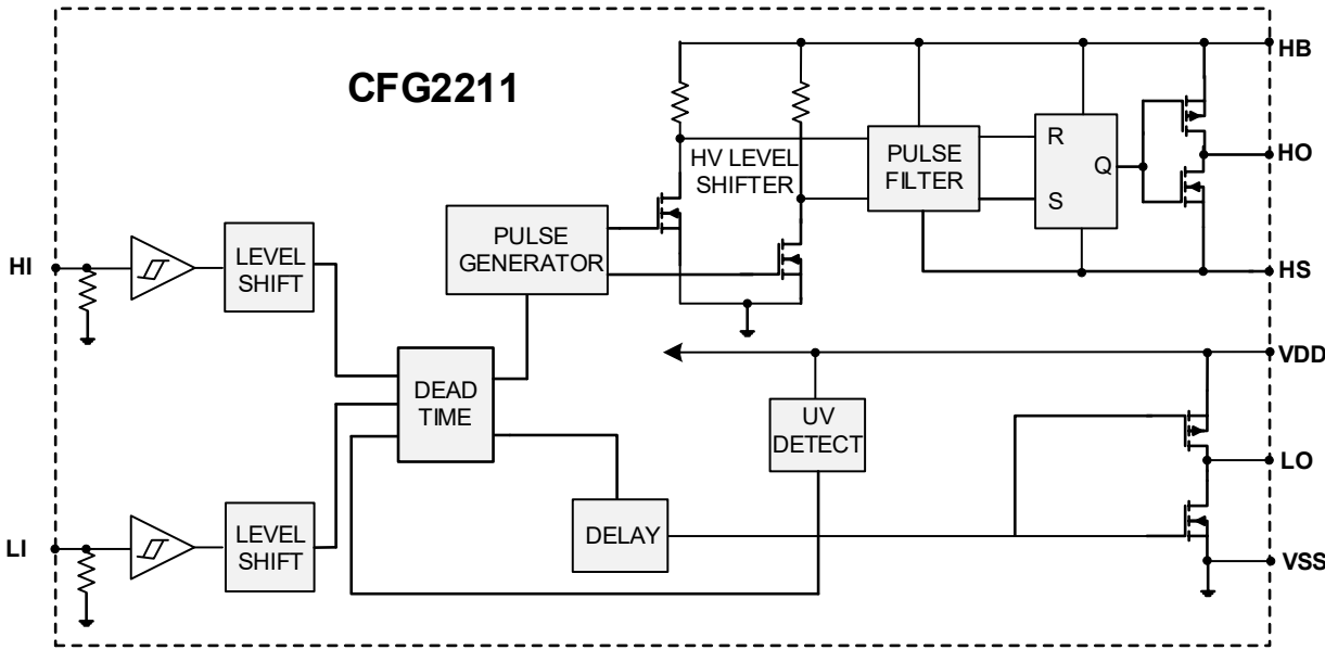
内部框图
