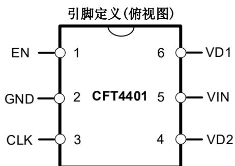
引脚功能
